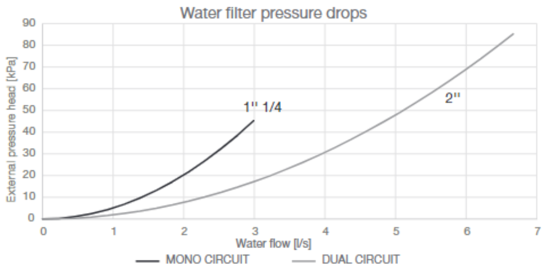
SI. 11 - Pad tlaka filtra za vodu
