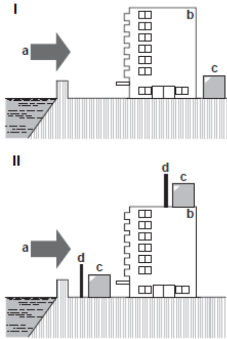
SI. 9 – Postavljanje vanjske jedinice uz moreSI
