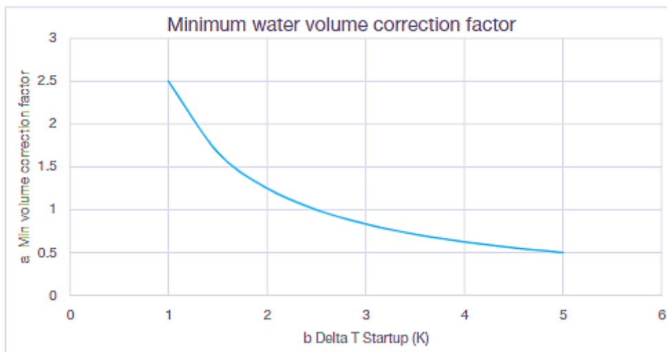
SI. 17 - Minimalni korekcijski faktor volumena vode
