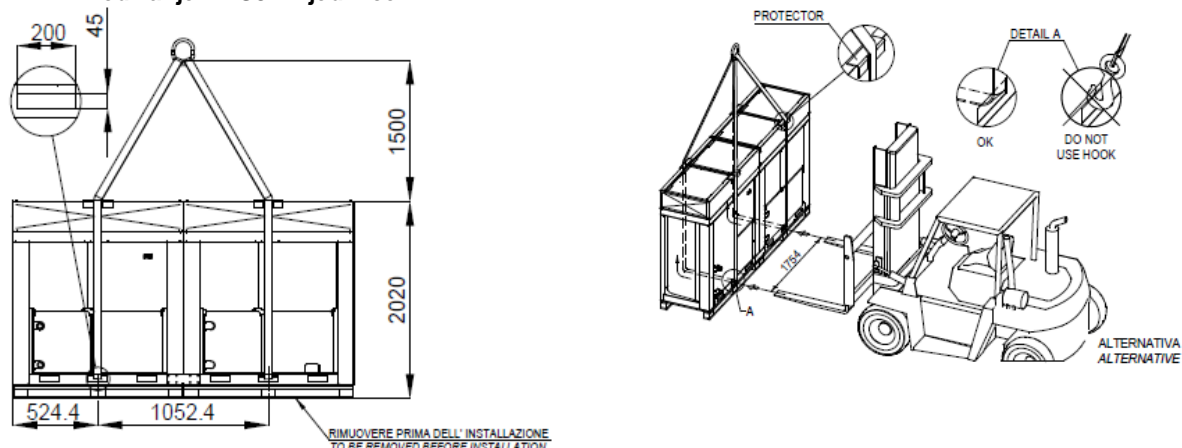
SI. 2 – Podizanje DVOJNE jedinice
