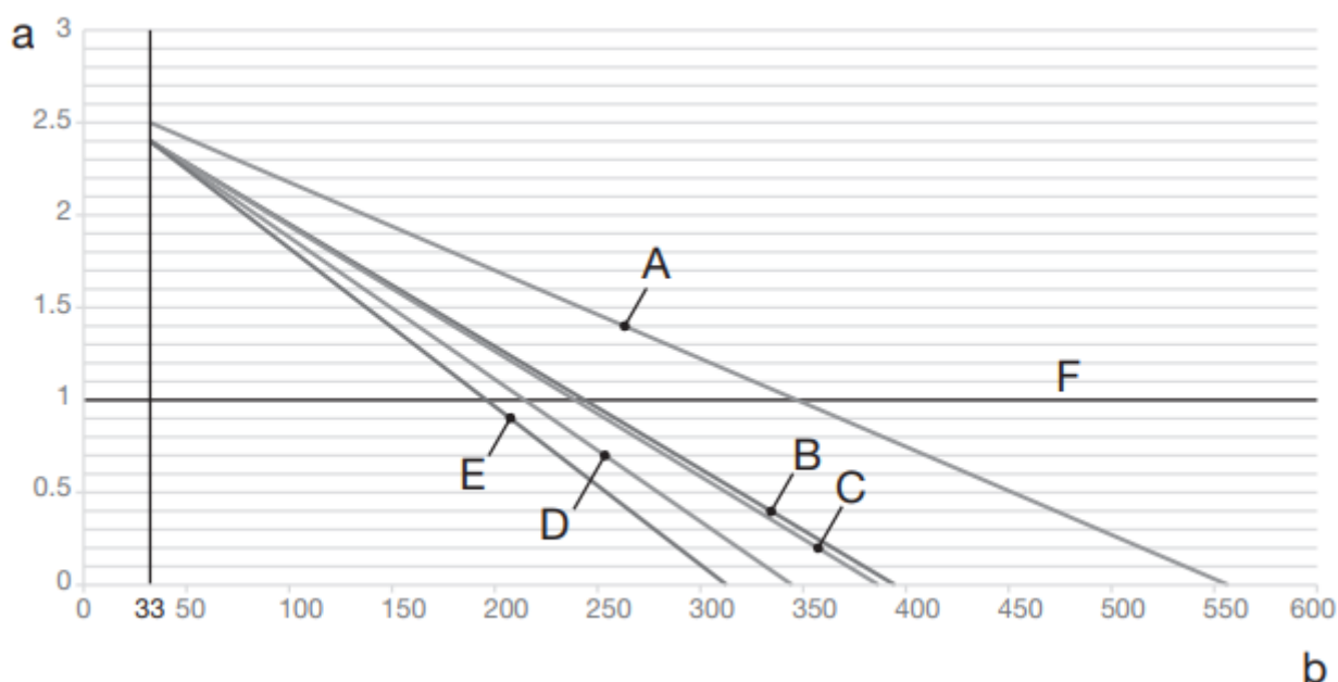
SI. 18 - Početni tlak ekspanzijske posude na temelju maksimalnog volumena vode
