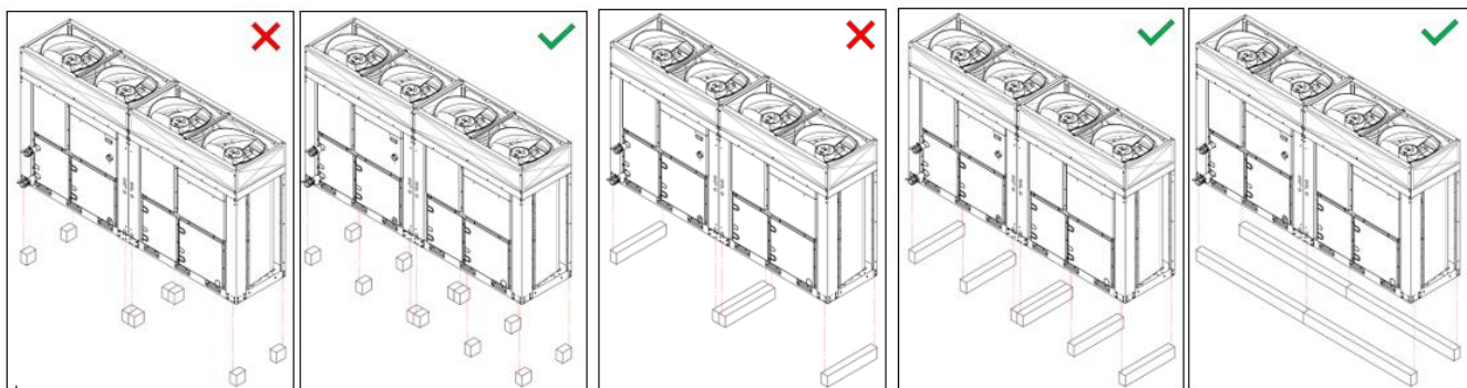
SI. 4 – Pozicioniranje DVOJNE jedinice
