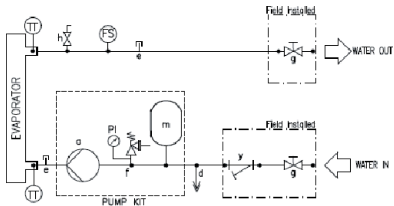
Sl. 10 – Hidraulički dijagrami
