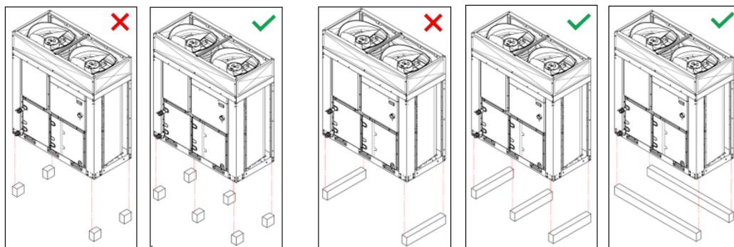
SI. 3 – Pozicioniranje MONO jedinice
