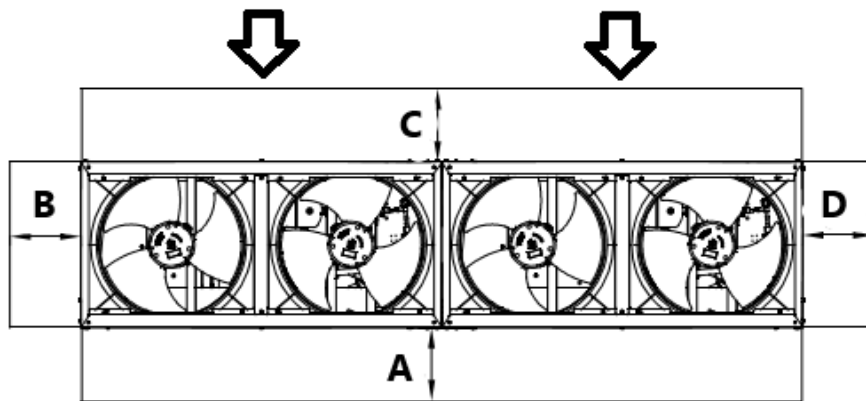
SI. 6 – DVOJNA JEDINICA
