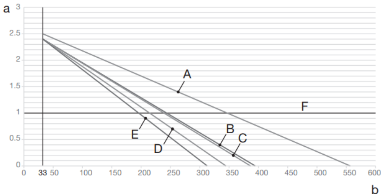
Figura 18 - Presión inicial del vaso de expansión tomando como base el volumen máximo de agua
