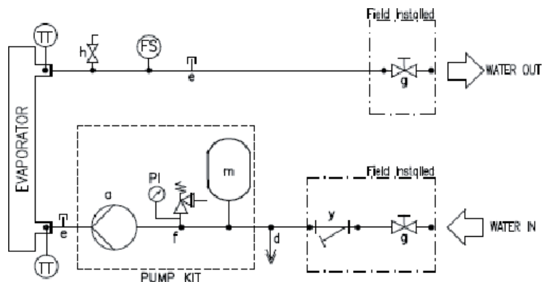
Figura 10 –Diagrama hidráulico
