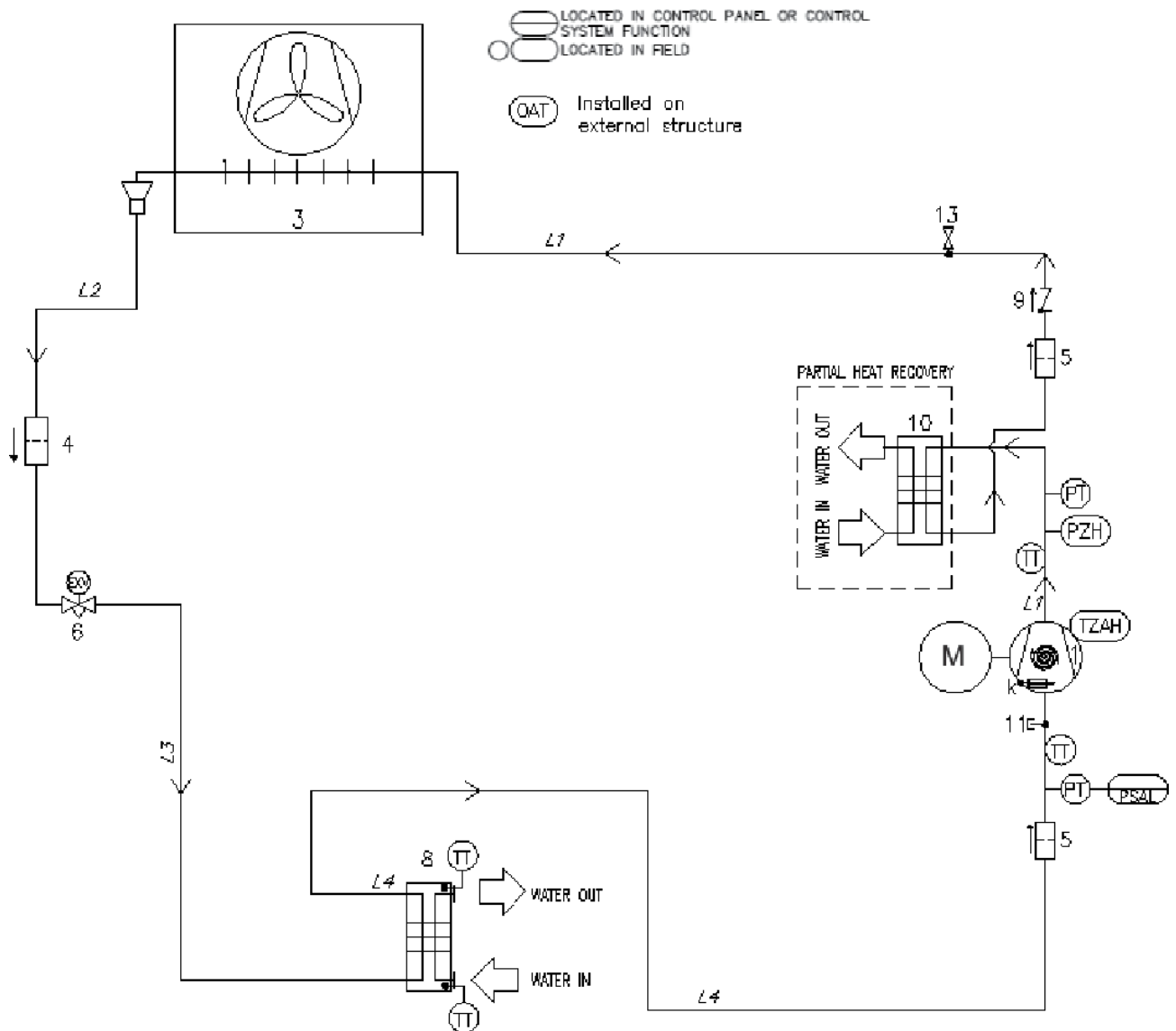
Figura 20 – Diagrama de circuito refrigerante (P&ID) para circuito MONO unidad EWAT-CZ
