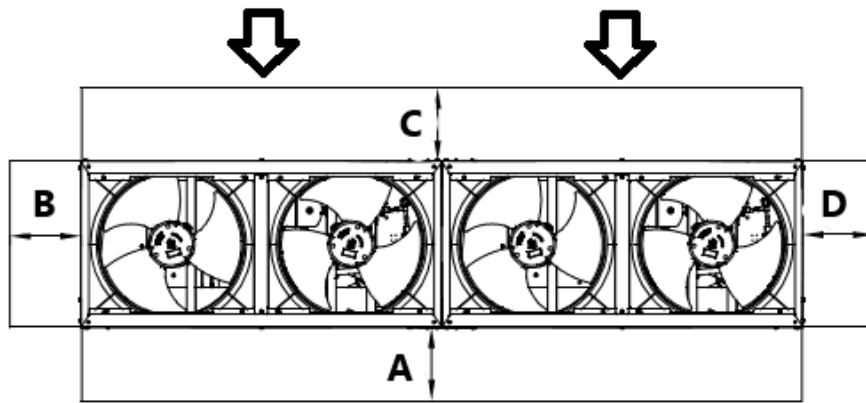
Figura 6 – Unidad DOBLE
