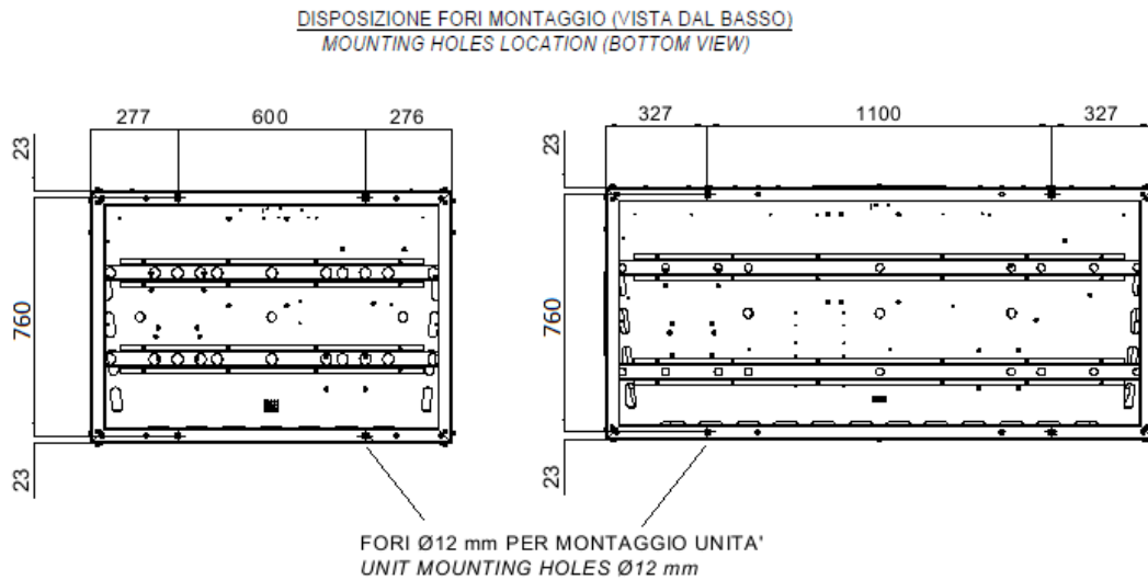
Figura 5 –Ubicación de los orificios de montaje (vista desde abajo)
