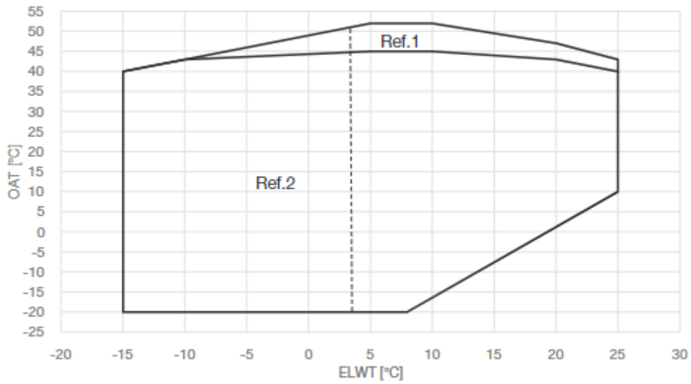
Figura 14 –Límites operativos en EWATCZ
