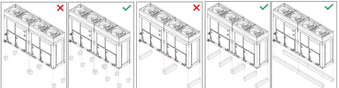
Figura 4 – Emplazamiento de la unidad DOBLE
