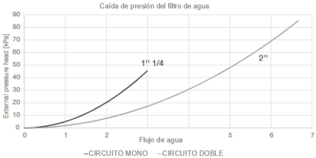
Figura 11 - Pérdidas de presión del filtro de agua
