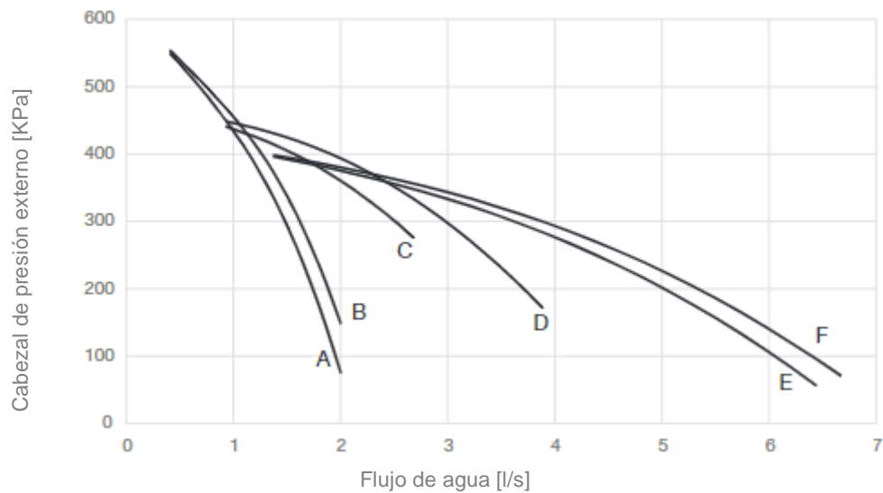
Figura 13 - Presión externa de bomba de elevación alta
