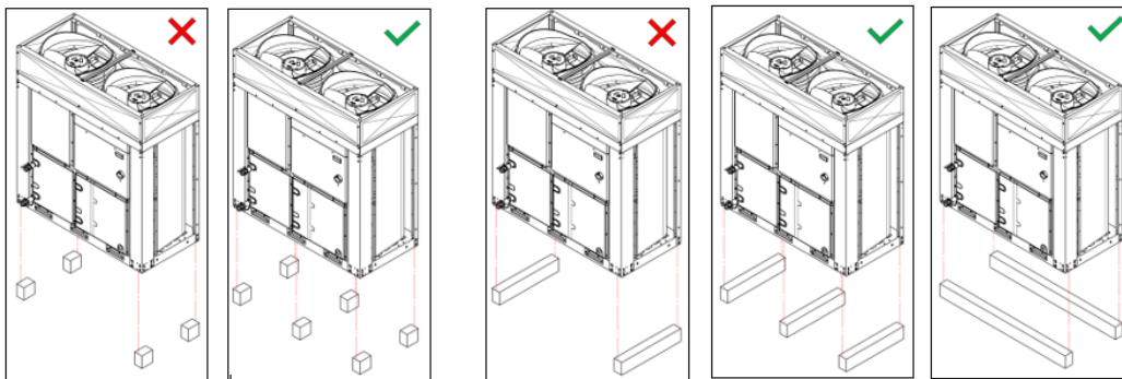
Figura 3 – Emplazamiento de la unidad MONO
