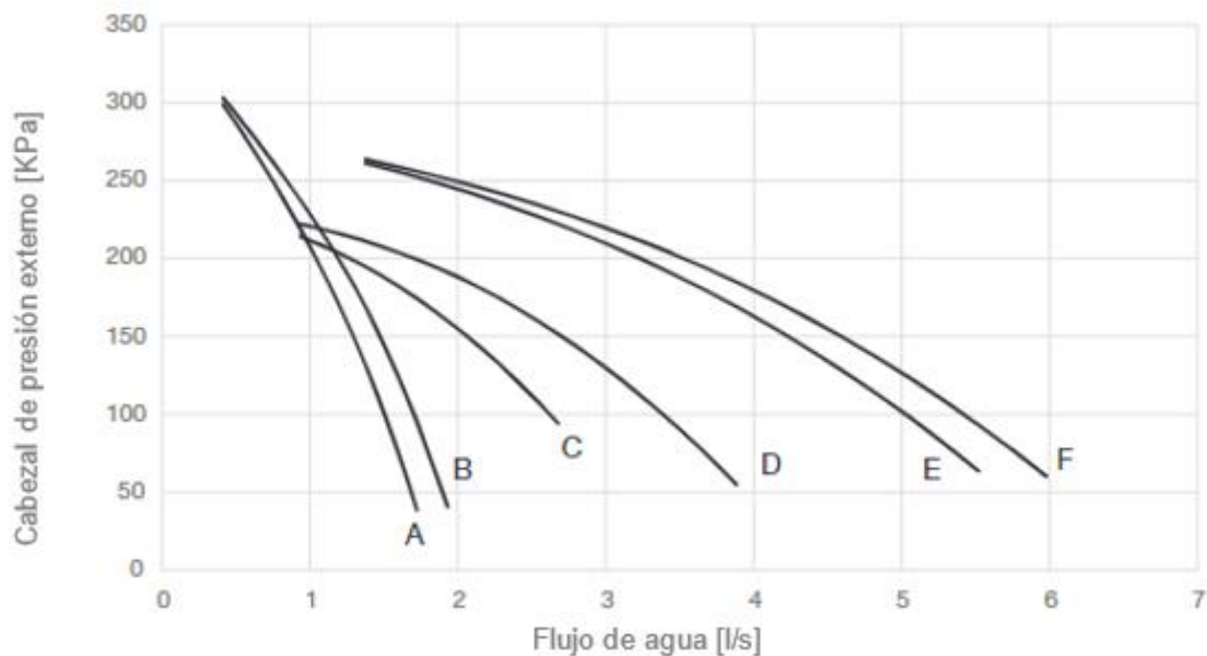
Figura 12 - Presión externa de bomba de elevación baja
