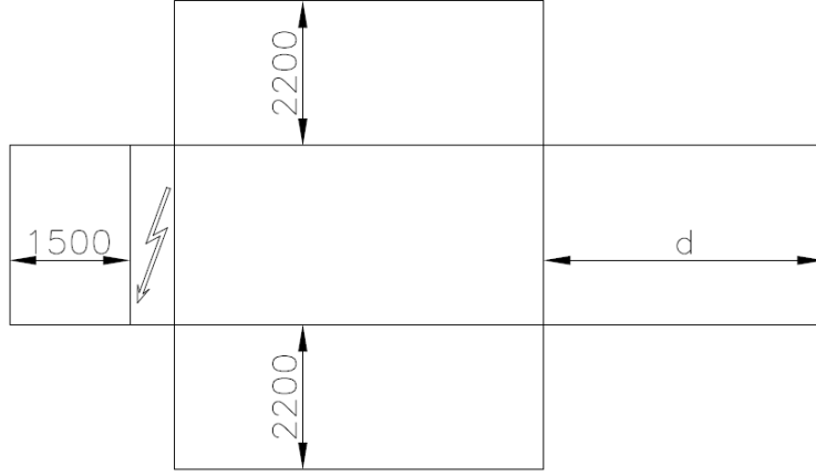
Şekil 5- Minimum açıklık gereksinimleri
