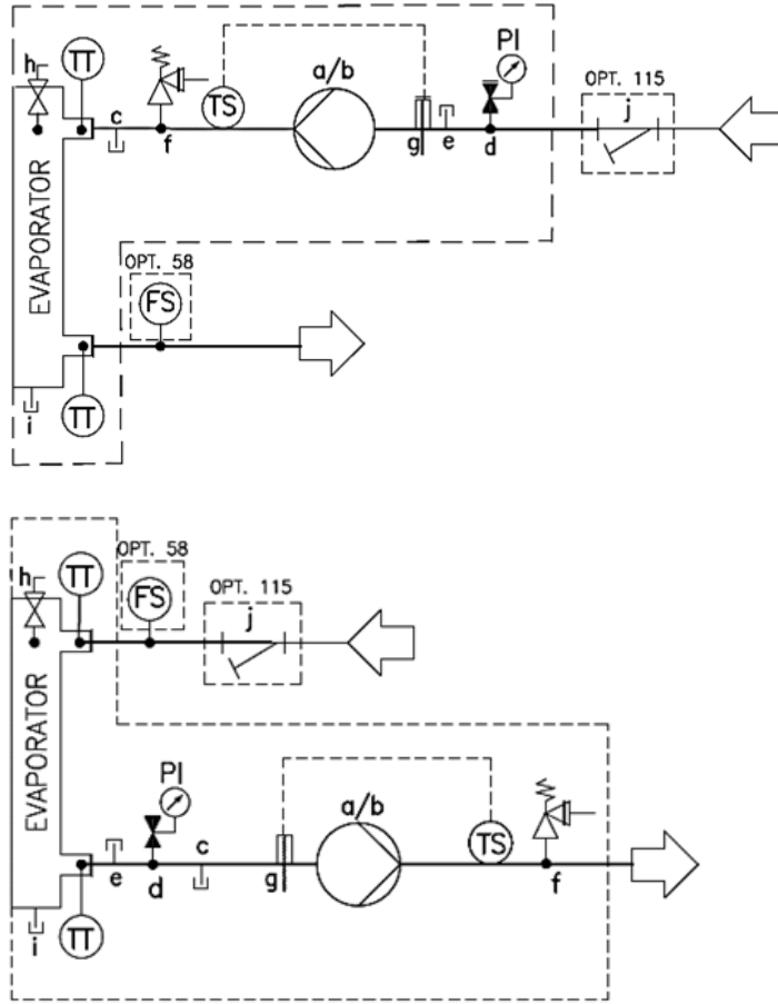
Şekil 7 - Evaporatör için su boru tesisatı bağlantısı (seçenekler 78-79-80-81)
