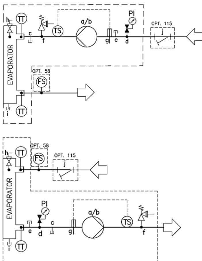
Afbeelding 7 - Aansluiting waterleiding voor verdamper (opt.78-79-80-81)
