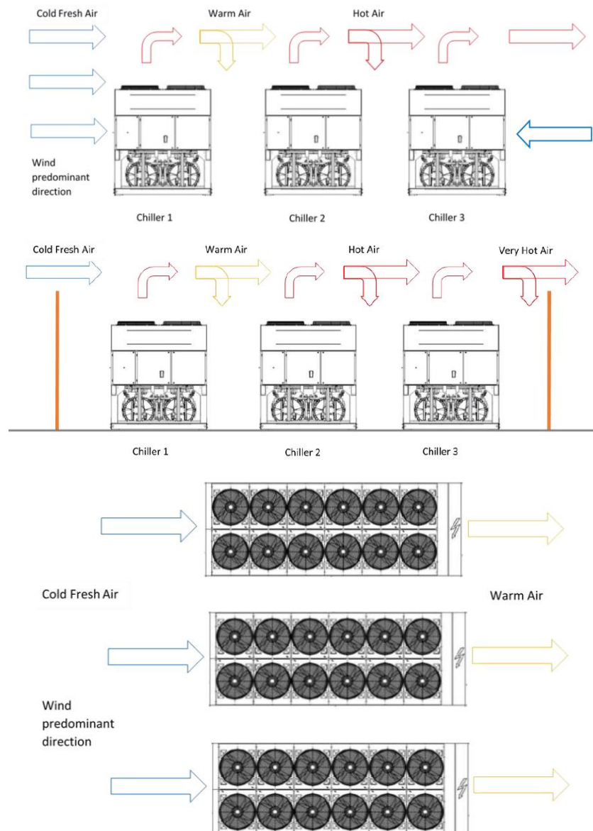
Afbeelding 6 – Installatie van meerdere koelers
