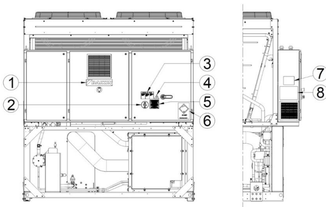
2. ábra - Az elektromos burokaltokra elhelyezett címkék értelmezése
