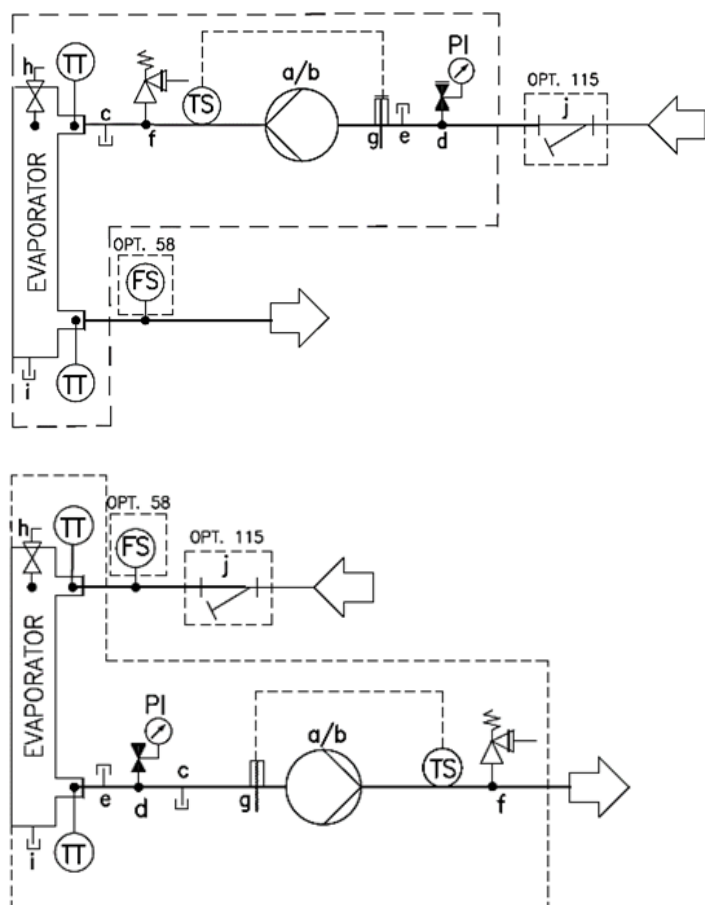
7. ábra - Vízvezeték-csatlakozás az elpárologtatóhoz (opt.78-79-80-81)
