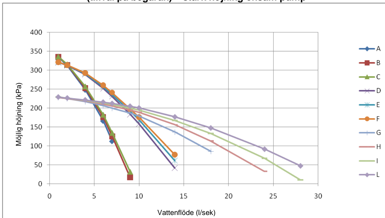
Figur 12 – EWAD E SS/SL – Tillgänglig extern höjning för sats med vattenpumpar (tillval på begäran) – stark höjning ensam pump
