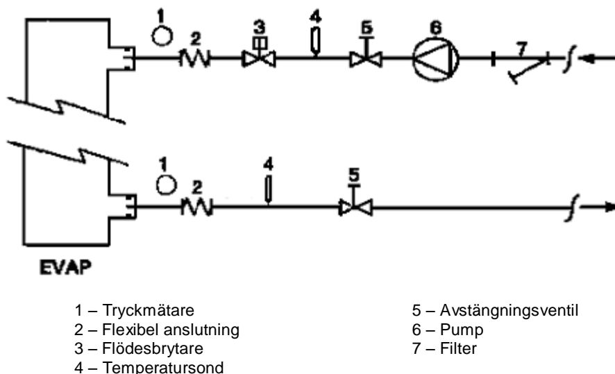
Figur 7 – Vattenledningsanslutningar till förångare
