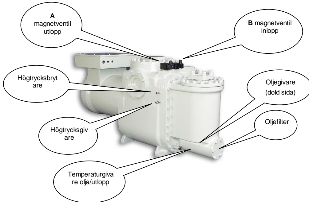
Figur 32 – Installation av styrenheter för kompressor Fr3100
