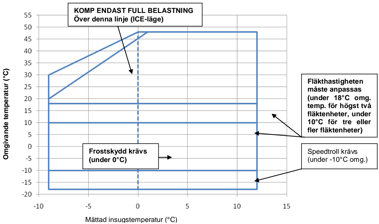
Figur 3 – Begränsningar vid drift – ERAD E-SS/SL
