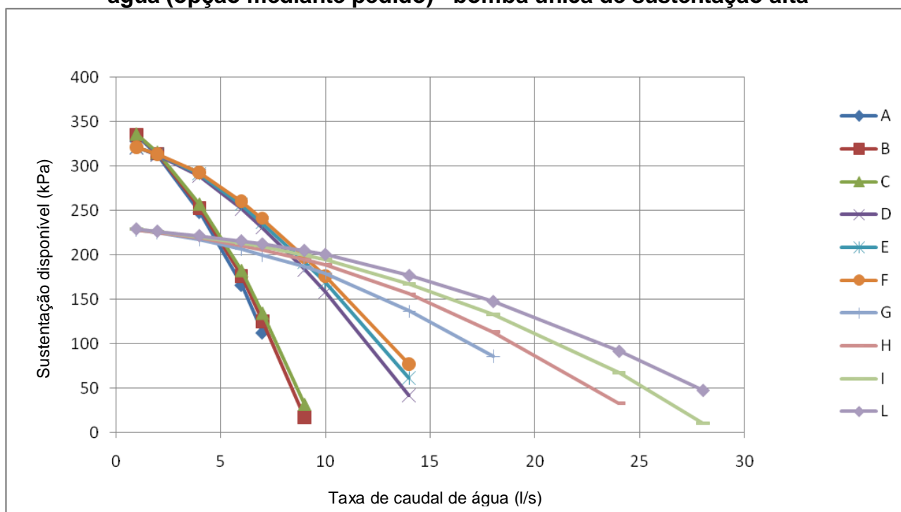
Figura 12 – EWAD E SS/SL - Elevador externo disponível para kit de bombas de água (opção mediante pedido) - bomba única de sustentação alta
