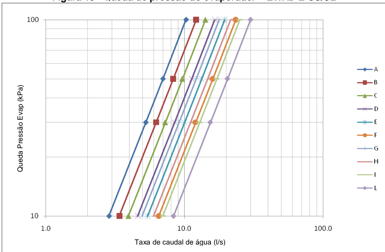
Figura 15 - Queda de pressão do evaporador – EWAD E-SS/SL
