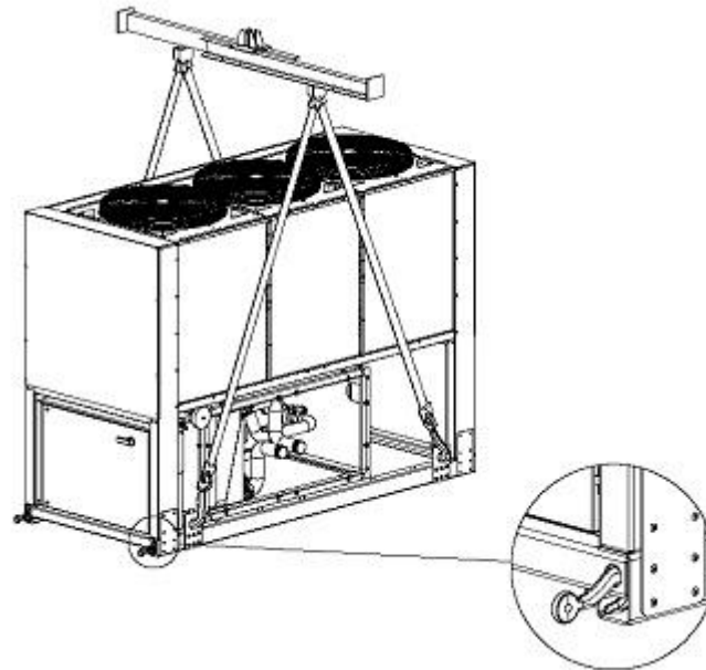
Procedimento de extração da unidade do contentor. (Kit contentor Opcional)
