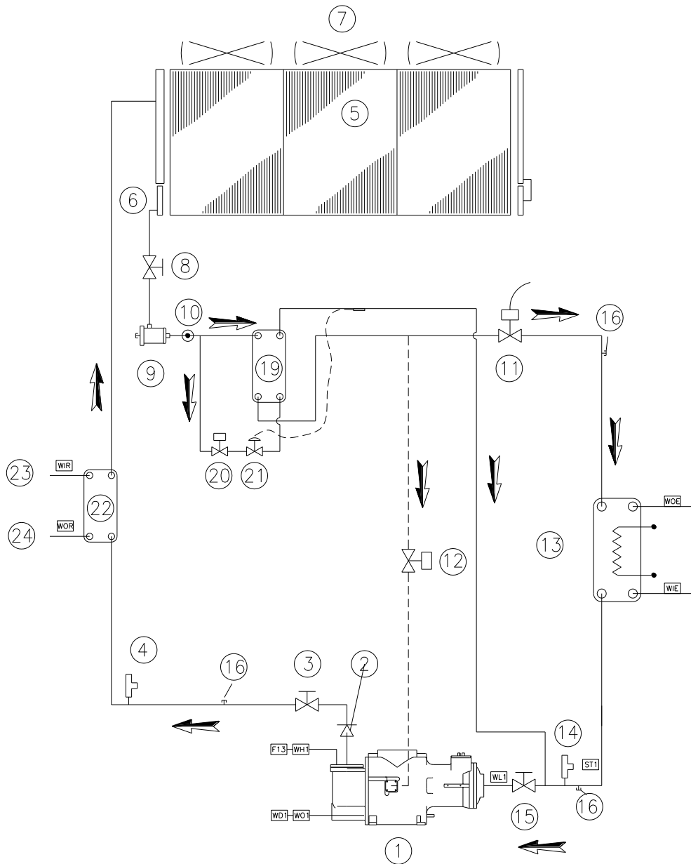
Figura 23 - EWAD 100E ÷ 410E SS – EWAD 100E ÷ 400E SL Circuito refrigerante do recuperador de calor - Unidades não economizadas
