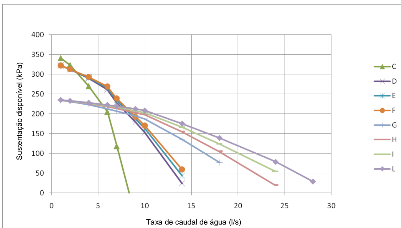
Figura 14 – EWAD E SS/SL - Elevador externo disponível para kit de bombas de água (opção mediante pedido) - bomba dupla de sustentação alta
